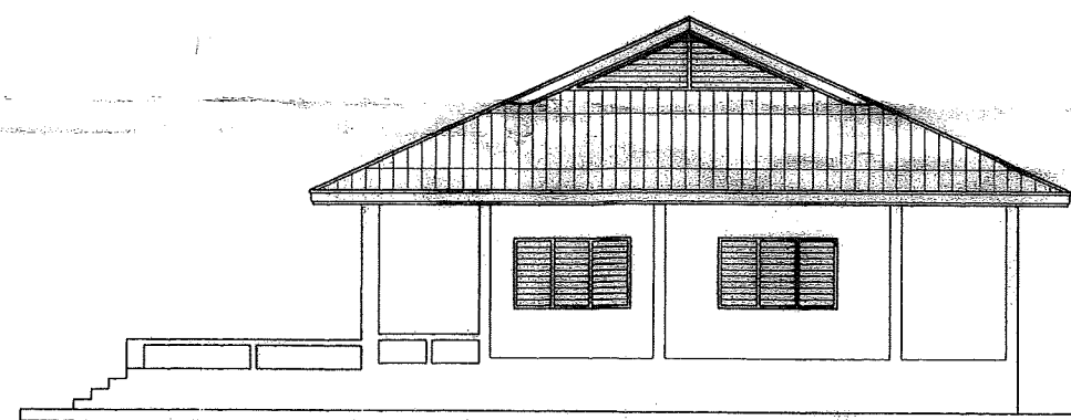
รูปด้าน ④ 1 : 100
