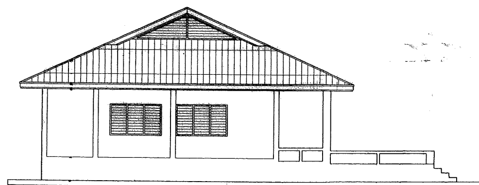
รูปด้าน ② 1 : 100
