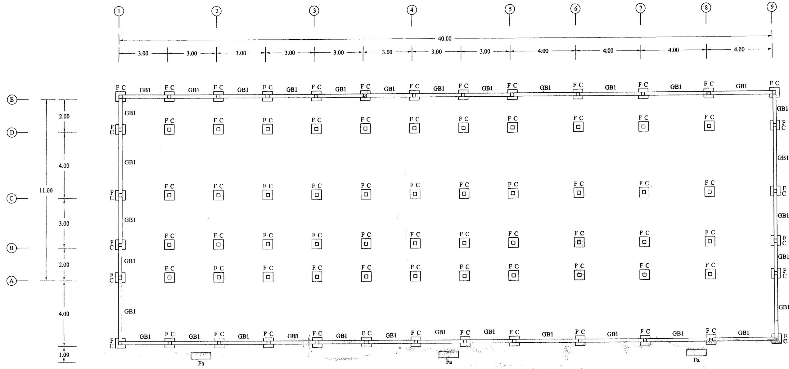
ผังฐานราก-คานคอดิน 1 : 100
