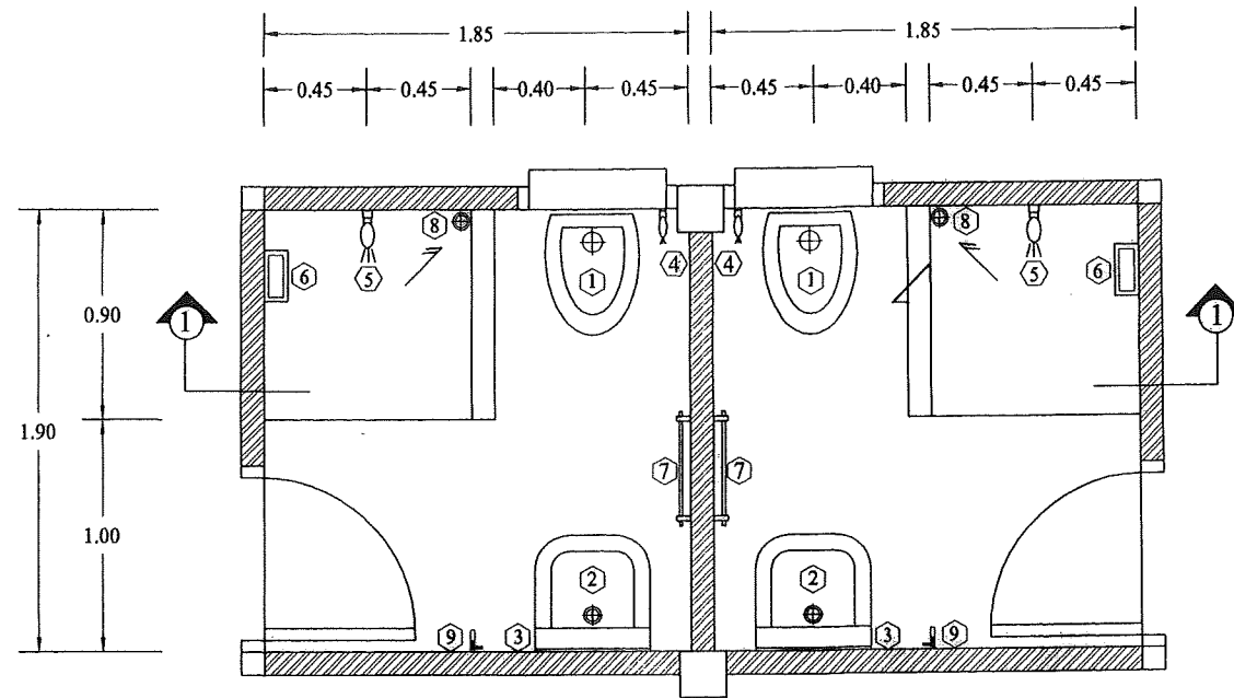
แปลนห้องน้ำ 1 1 : 25
