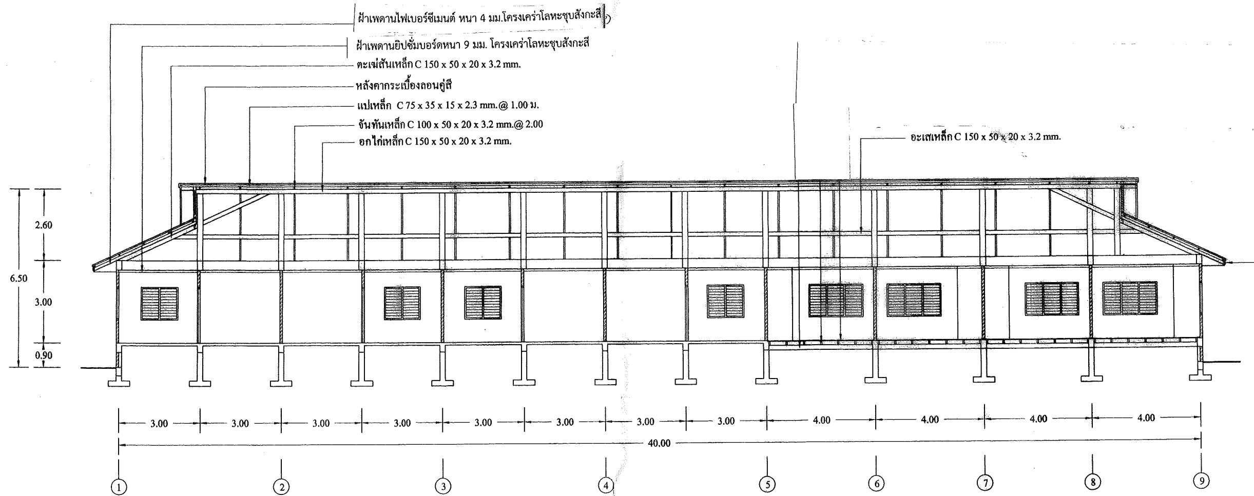
รูปตัด ①-① 1 : 100
