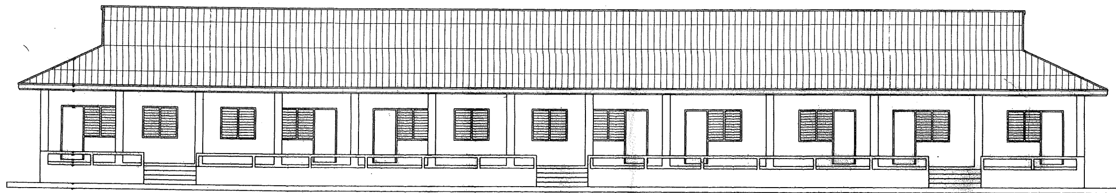
รูปด้าน ① 1 : 100
