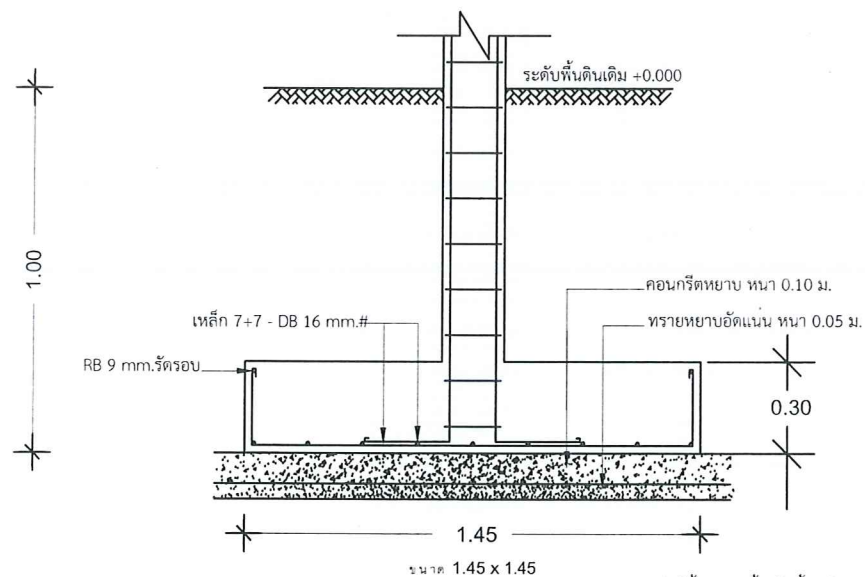
ขยายรูปตัดฐานราก F มาตราส่วน 1: 25
