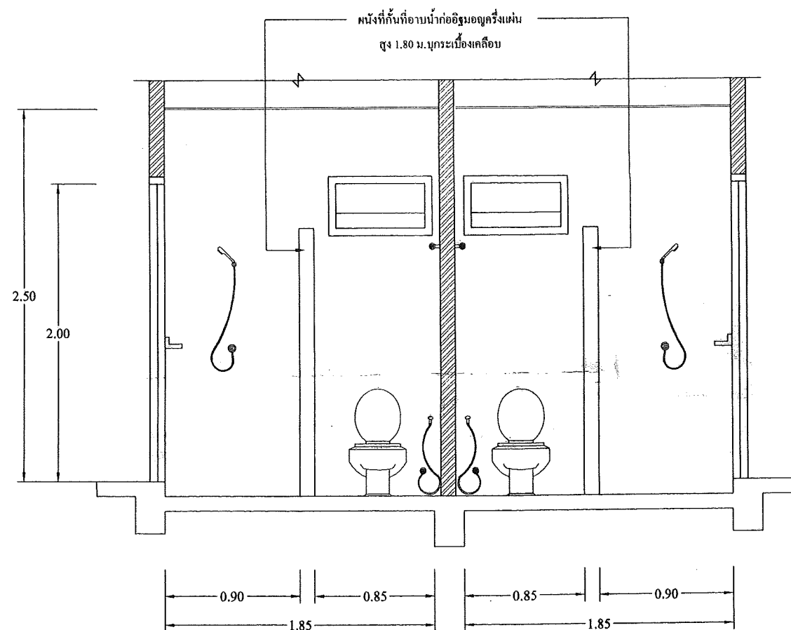
รูปตัด 1-1 1 : 25
