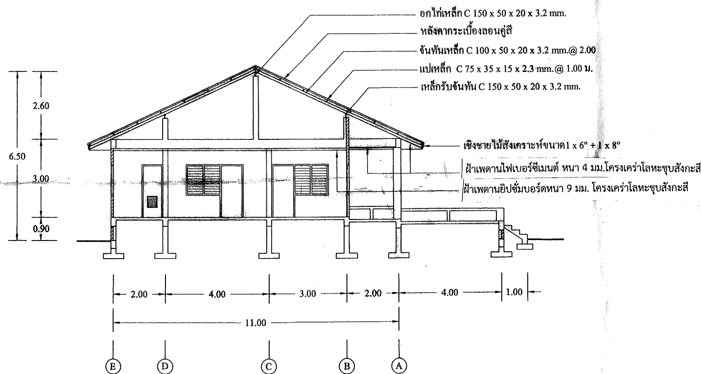
รูปตัด ①-① 1 : 100
