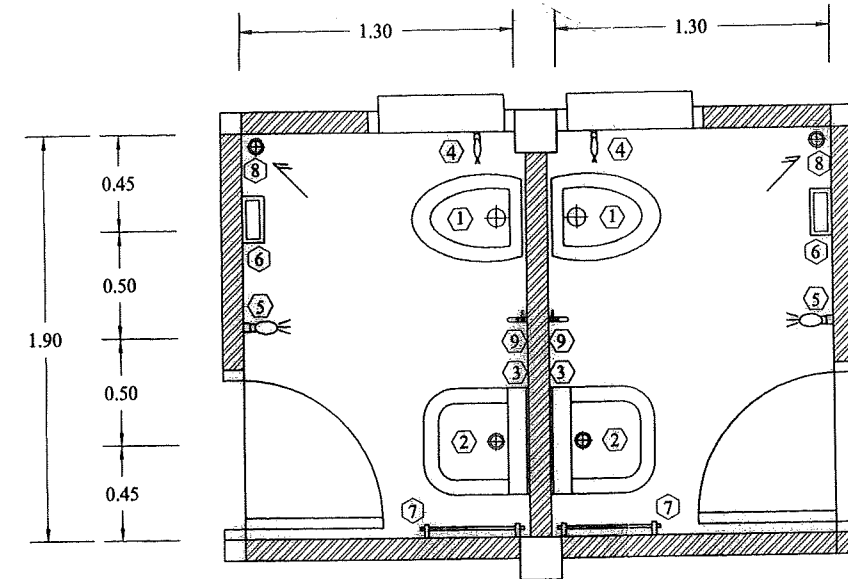
แปลนห้องน้ำ 2 1 : 25
