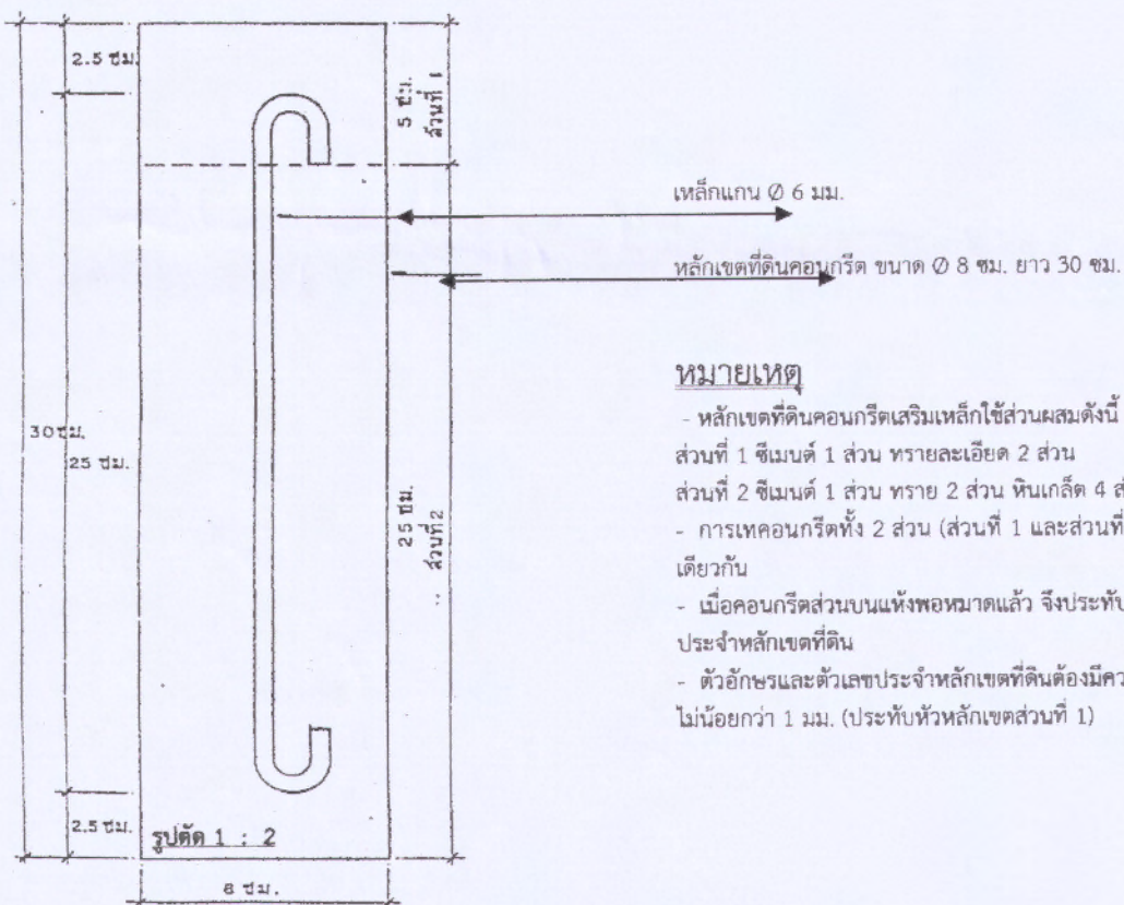
รูปตัด Scale 1 : 2
