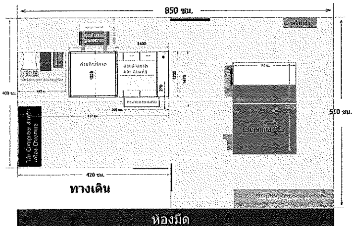
แผนผังห้องสำหรับติดตั้งชุดเครื่องมืออัตโนมัติ ย่อ ขยาย ล้างภาพดิจิทัล
