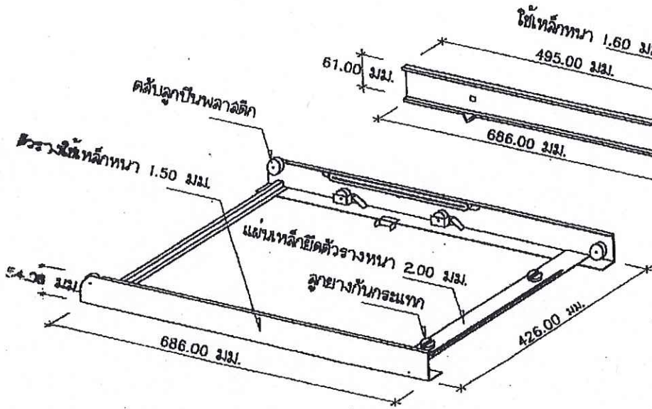
รูปขยาย D แสดงรางรองรับลิ้นชัก
