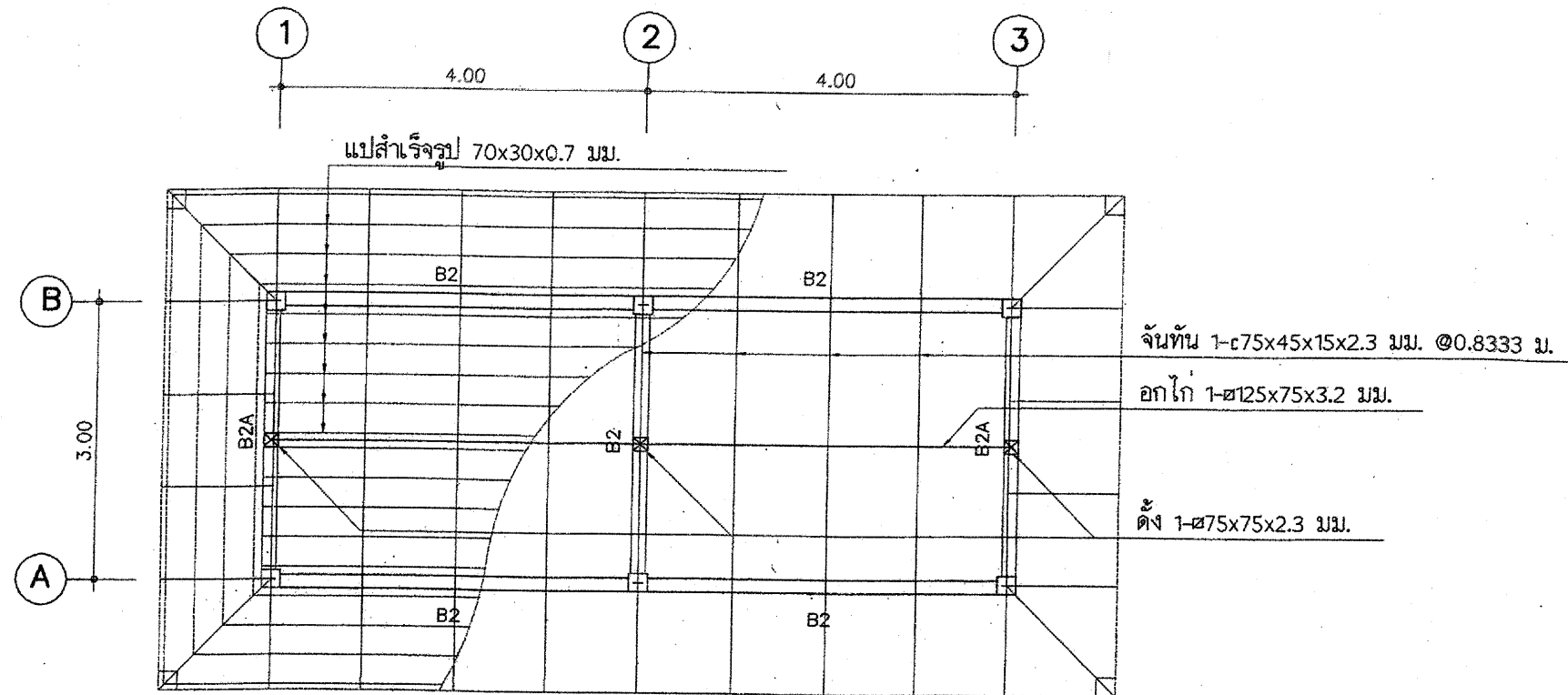
แปลนคาน และโครงสร้างหลังคา มาตรฐาน 1:75
