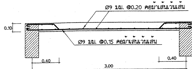
B2A 1:25
