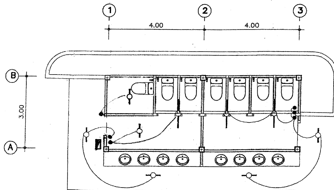
แปลนไฟฟ้า มาตรฐาน 1:100
