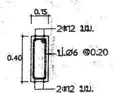
B2 1:25
