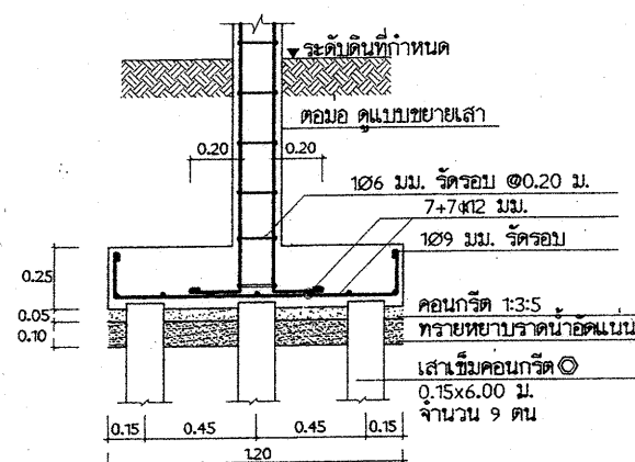
2-2 1:25
