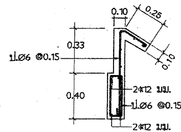
B2A 1:25
