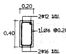
B3 1:25
