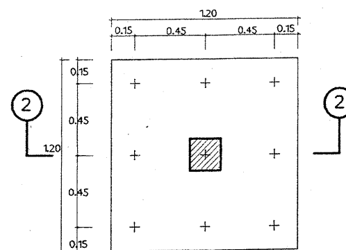
F2 1:25
