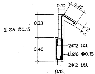
B2A 1:25
