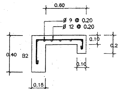
แบบขยายคานเตอร์
