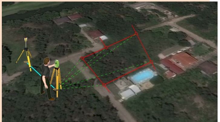
การโยงยึดหลักเขตที่ดิน
