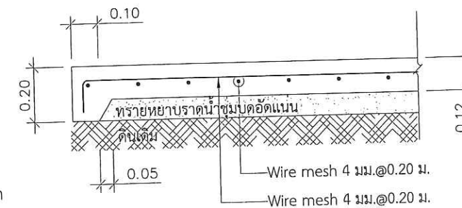
รูปขยายพื้น GS1 มาตราส่วน NTS
